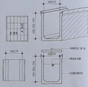
DET. SALURAN AIR Skala 1:50
