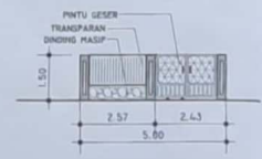
PAGAR Skala 1:100
