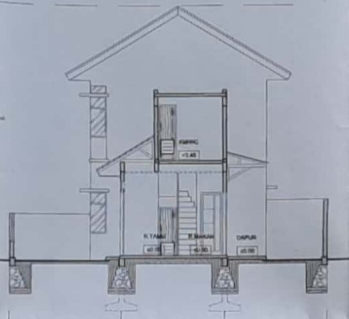
POTONGAN B-B Skala 1:100
