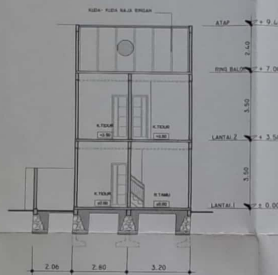
POTONGAN A-A Skala 1:100
