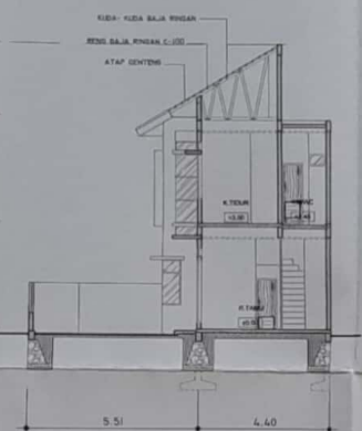
POTONGAN B-B Skala 1:100
