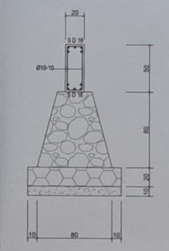
DET. BAK SAMPAH Skala 1:50
