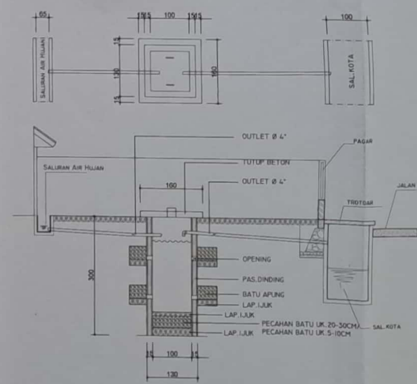
DET. S. RESAPAN Skala 1:50
