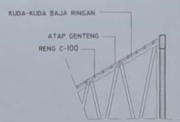
DET. KUDA-KUDA Skala 1:50
